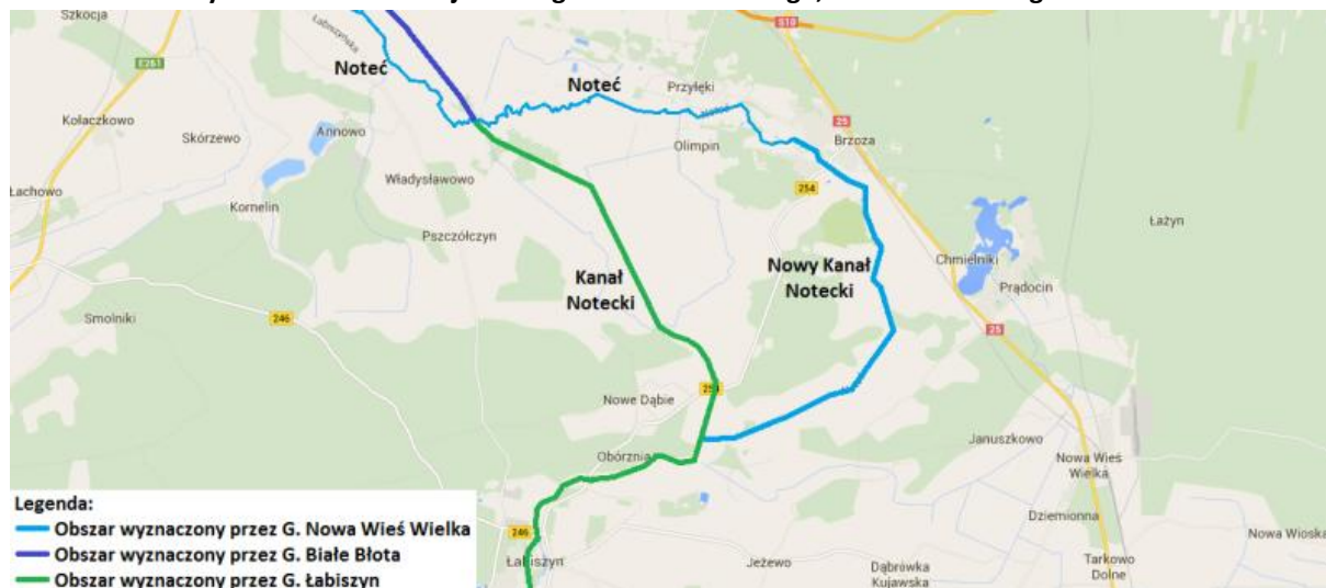
Rysunek 29. Lokalizacja Nowego Kanału Noteckiego, Kanału Noteckiego i Noteci
